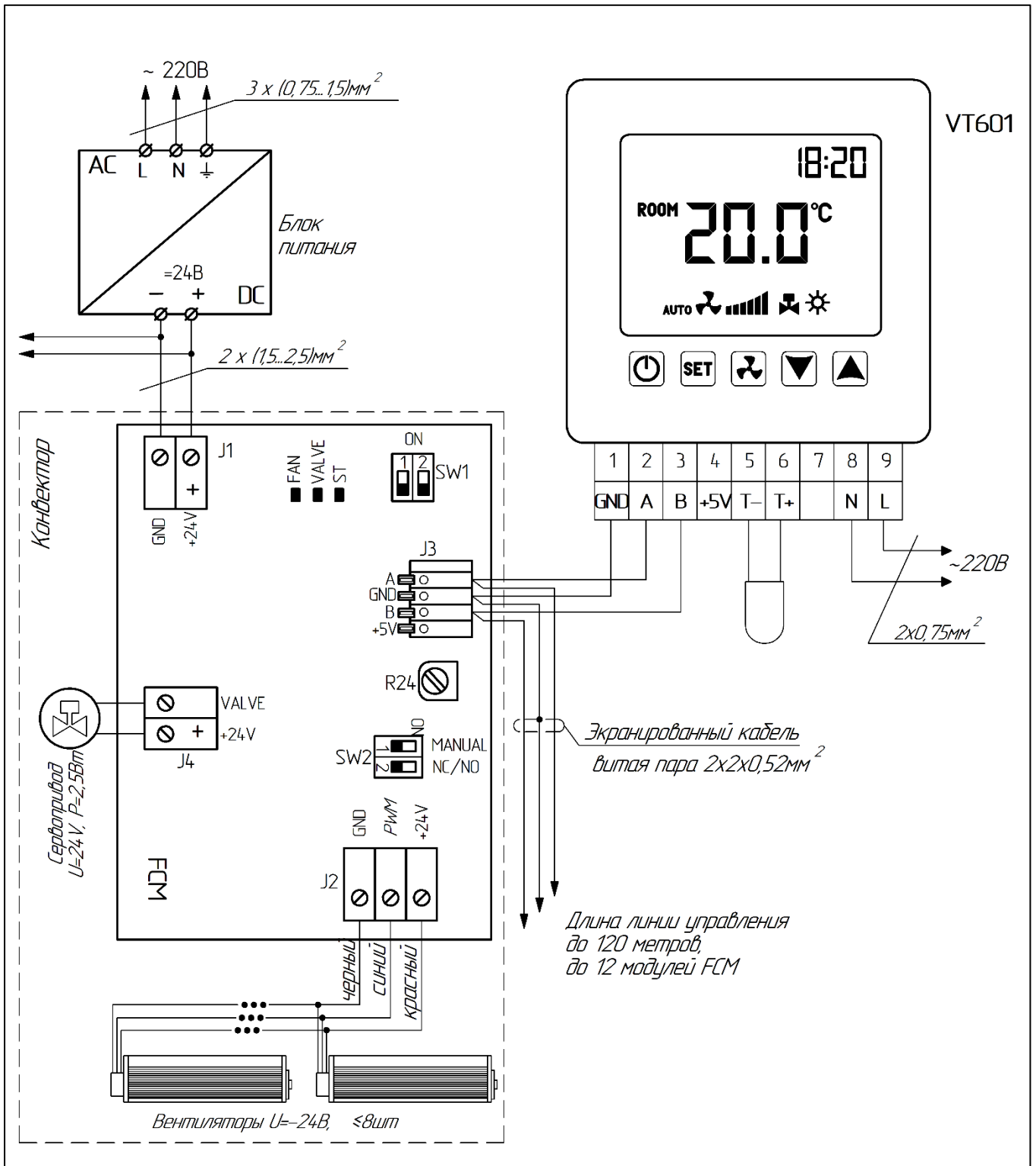
Схема соединений для Брыз В НЕРЖ 24В (вентиляторы 24В постоянного тока с ШИМ-управлением).
